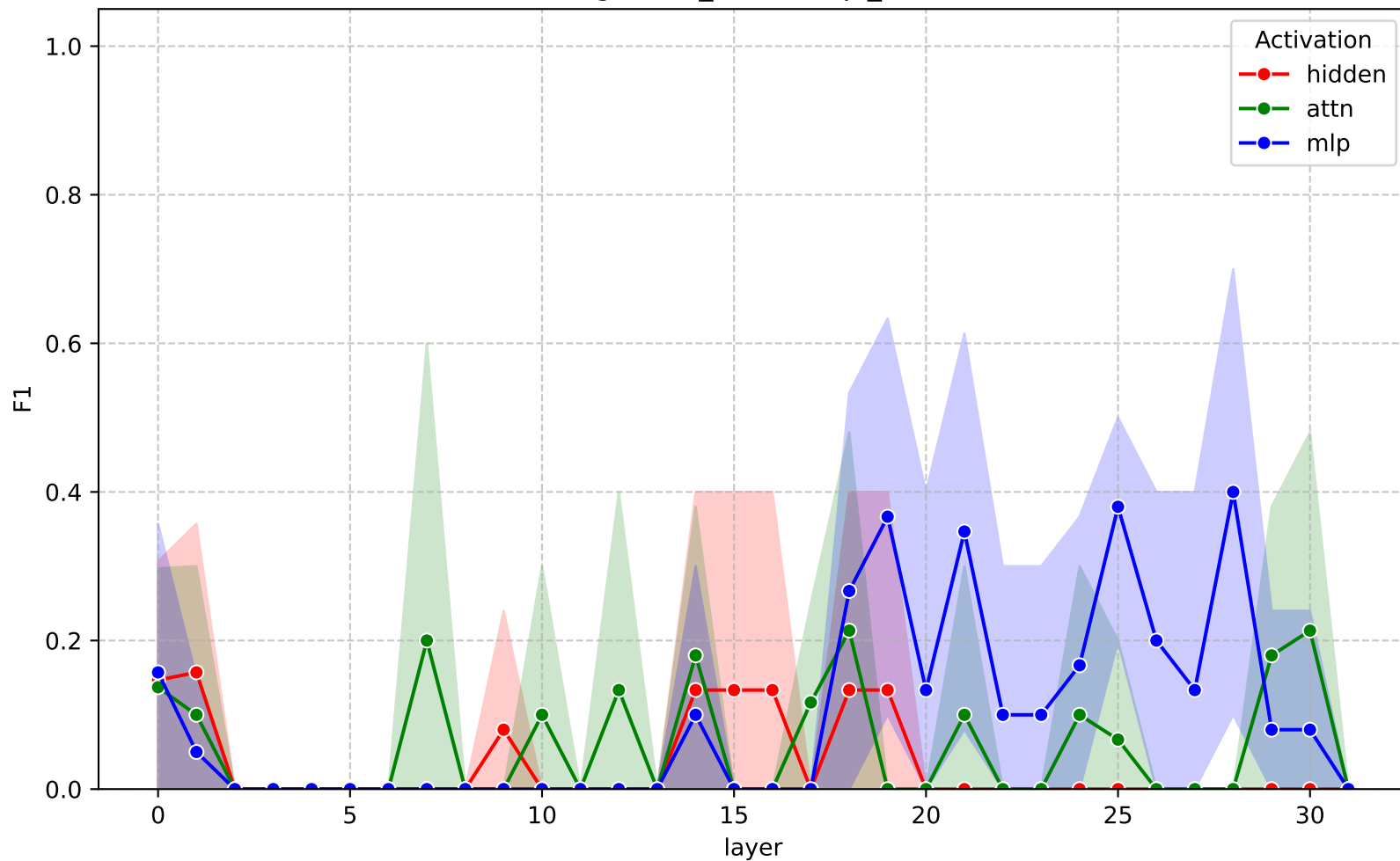
F1 across layers - gemma-3-4b-it (ragbench_delucionqa_svm)
