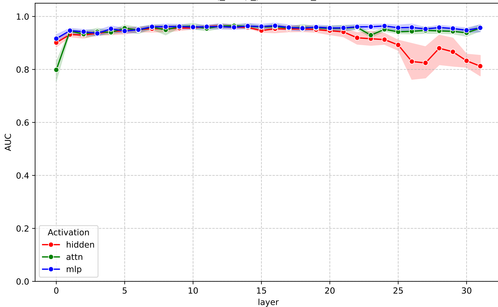
AUC across layers - gemma-3-4b-it (nq_swap_parametric_ffn)
