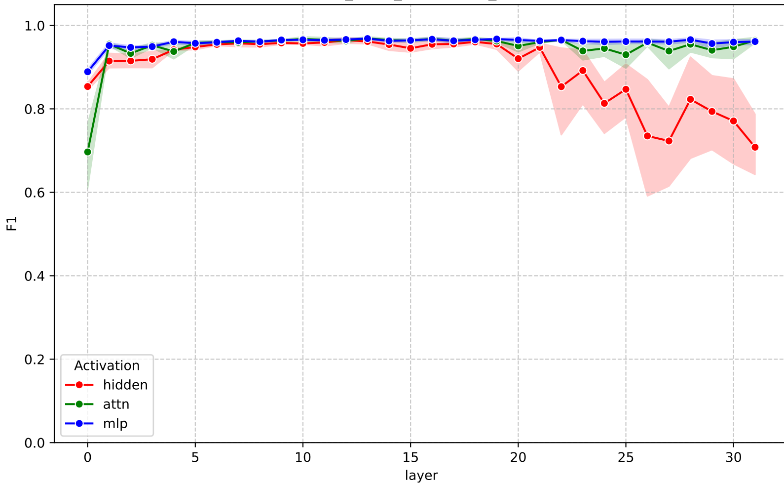
F1 across layers - gemma-3-4b-it (nq_swap_parametric_ffn)
