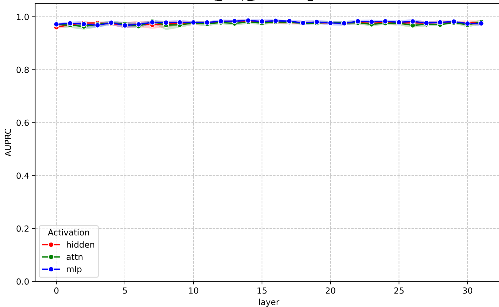
AUPRC across layers - gemma-3-4b-it (nq_swap_parametric_svm)
