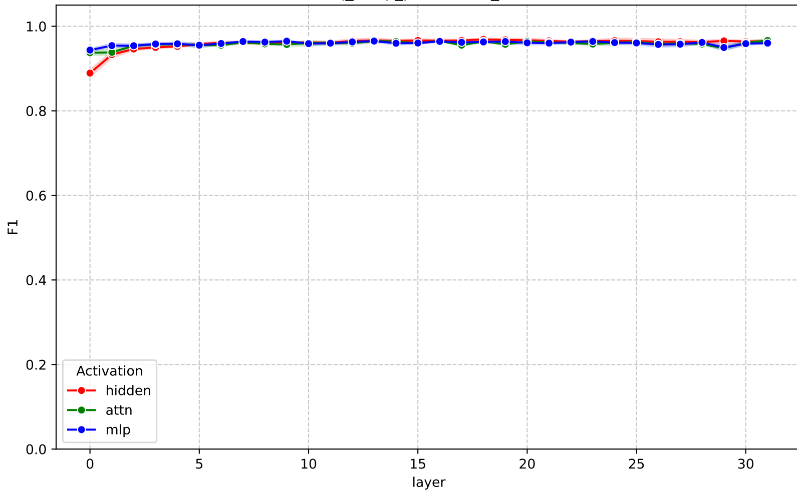
F1 across layers - gemma-3-4b-it (nq_swap_parametric_svm)
