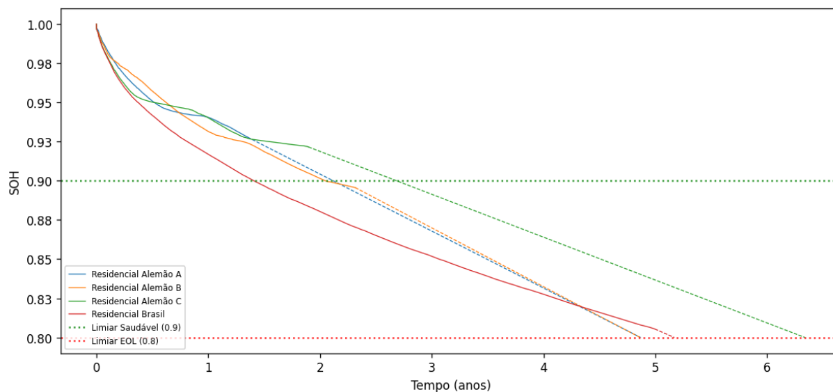
Gráfico 3 - Comparação da evolução do SOH entre perfis residenciais
