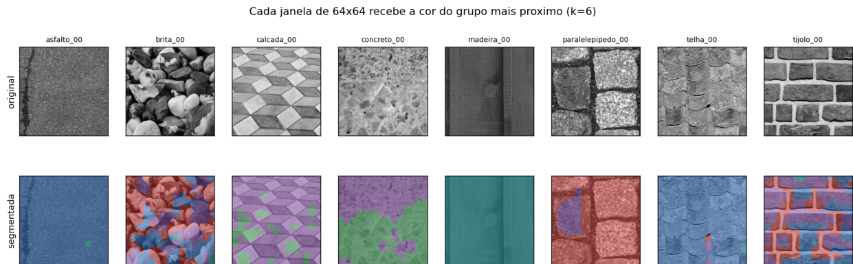
Figura 3. Acima as originais, abaixo o mapa de grupos sobreposto. Em tijolo_00 as juntas de argamassa saem em laranja, separadas das faces dos tijolos; em paralelepipedo_00 uma pedra de granulação diferente se destaca das vizinhas; em concreto_00 as duas regiões de granulação distinta são separadas.
