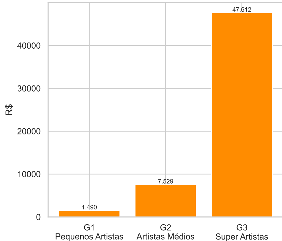
MAE no teste (R$)
