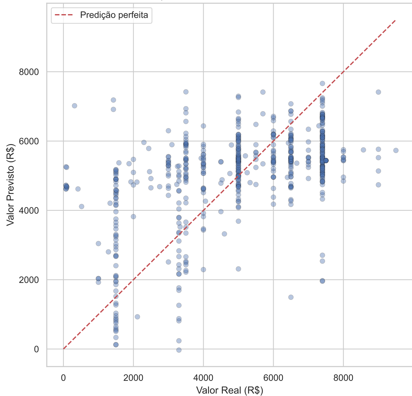
G1 — Pequenos Artistas — Teste: Real vs. Previsto
