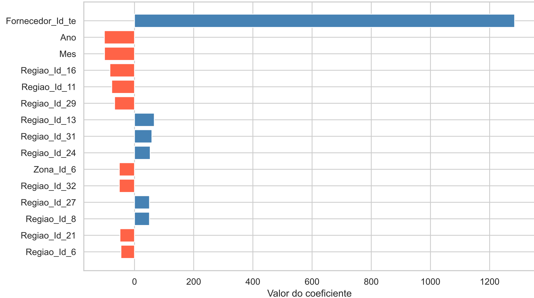
G1 — Pequenos Artistas — Top 15 coeficientes da Regressão Linear
