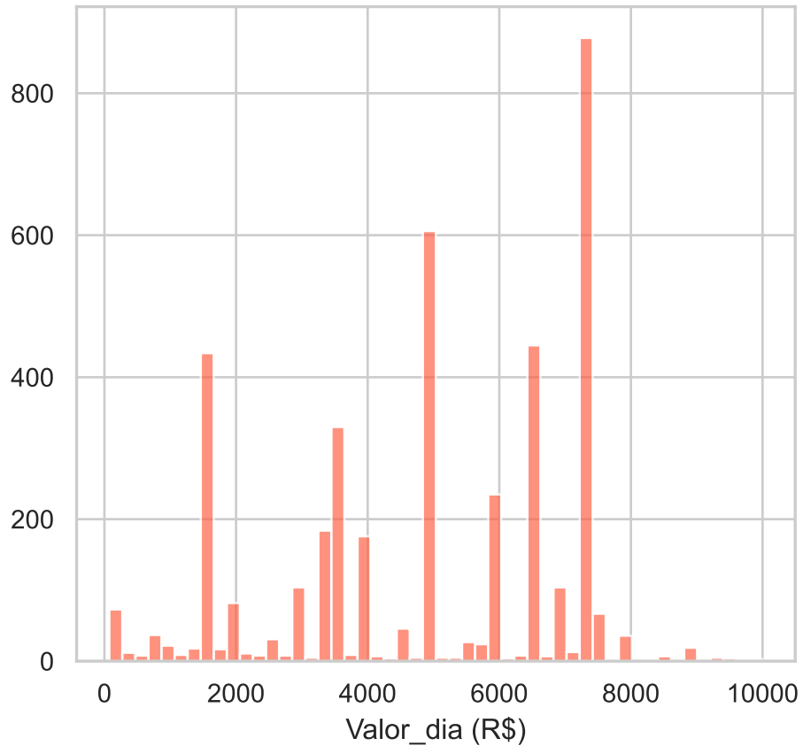
G1 — Pequenos Artistas — Valor_dia ANTES do tratamento
