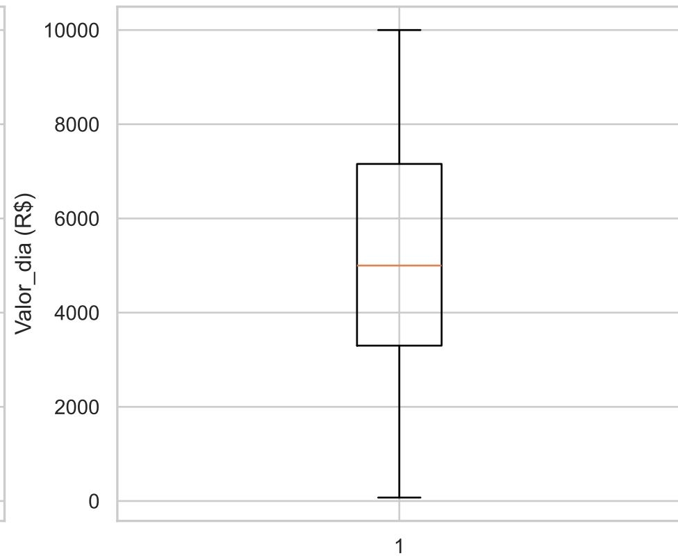
G1 — Pequenos Artistas — Valor_dia SEM anomalias IQR
