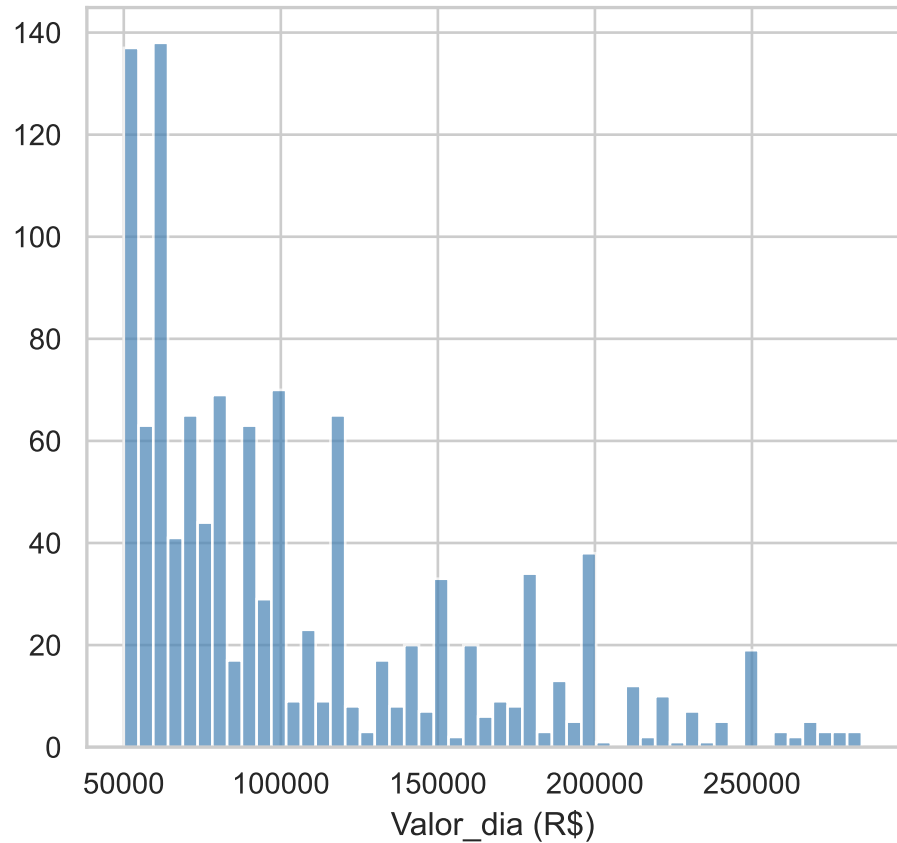
G3 — Super Artistas — Valor_dia DEPOIS do tratamento
