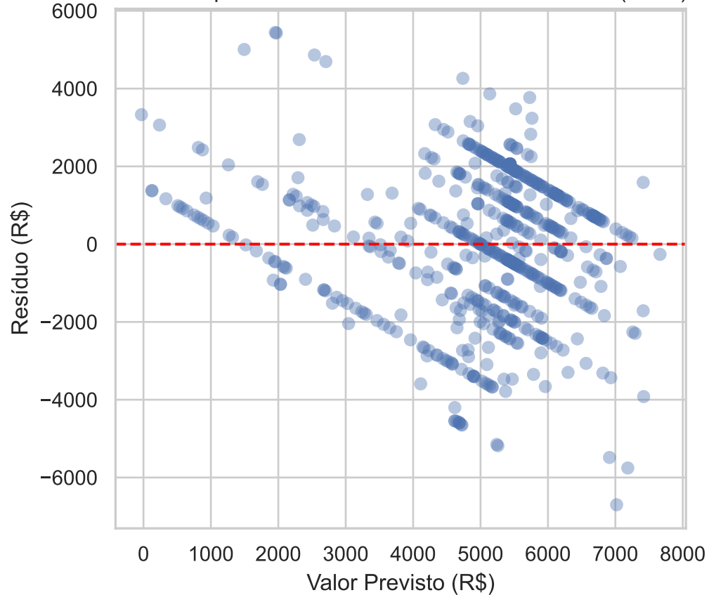
G1 — Pequenos Artistas — Resíduos vs. Previsto (Teste)
