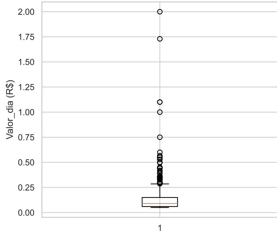
1e6 G3 — Super Artistas — Valor_dia COM anomalies
