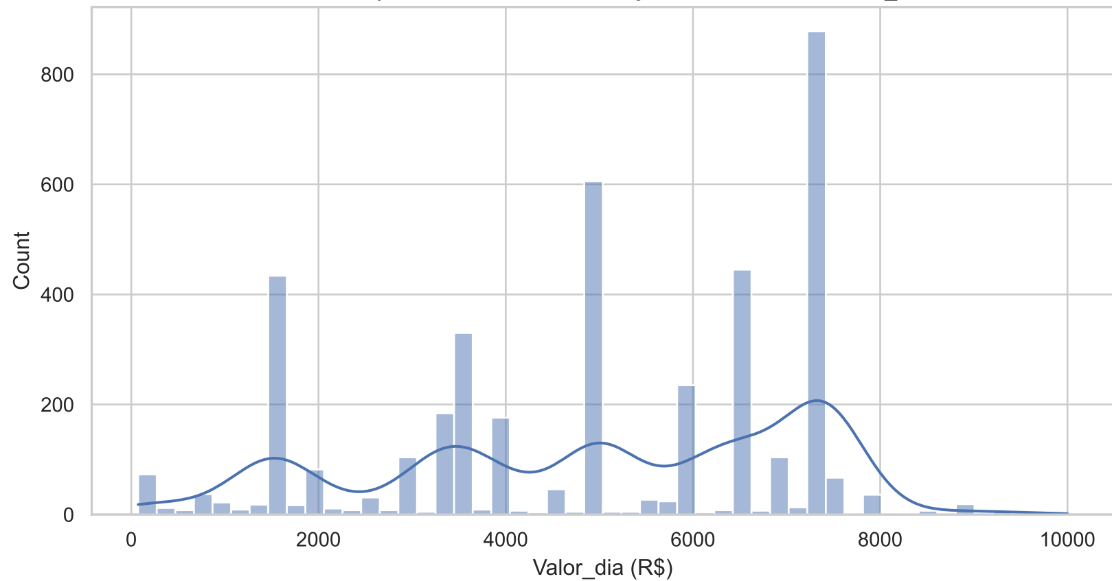
G1 — Pequenos Artistas — Distribuição da variável-alvo Valor_dia
