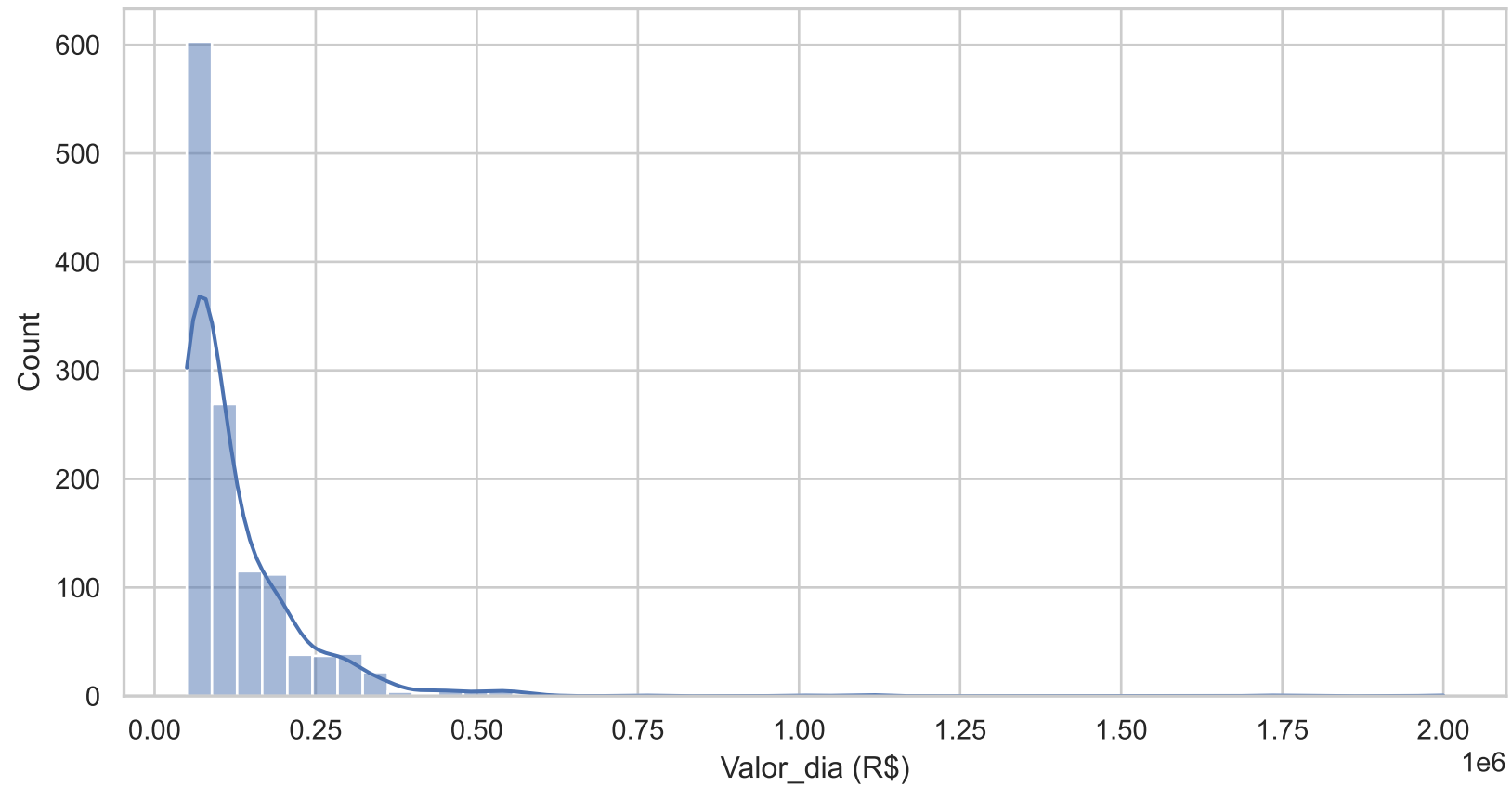
G3 — Super Artistas — Distribuição da variável-alvo Valor_dia
