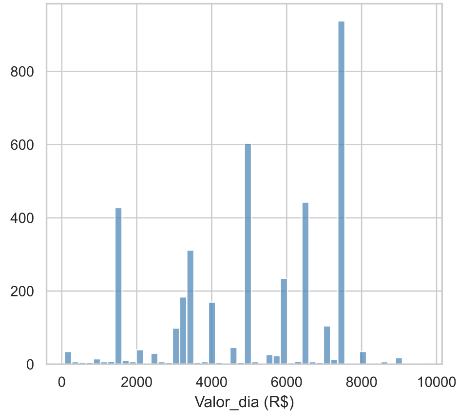
G1 — Pequenos Artistas — Valor_dia DEPOIS do tratamento
