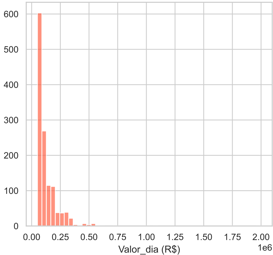
G3 — Super Artistas — Valor_dia ANTES do tratamento
