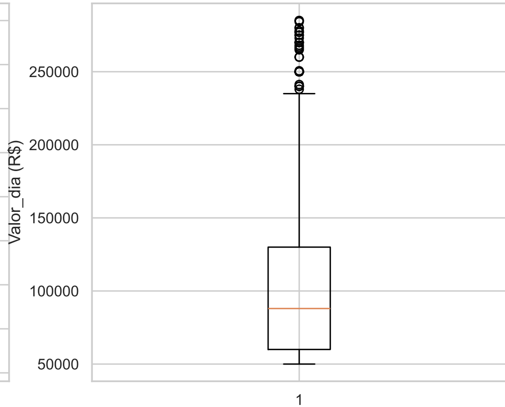
G3 — Super Artistas — Valor_dia SEM anomalies IQR
