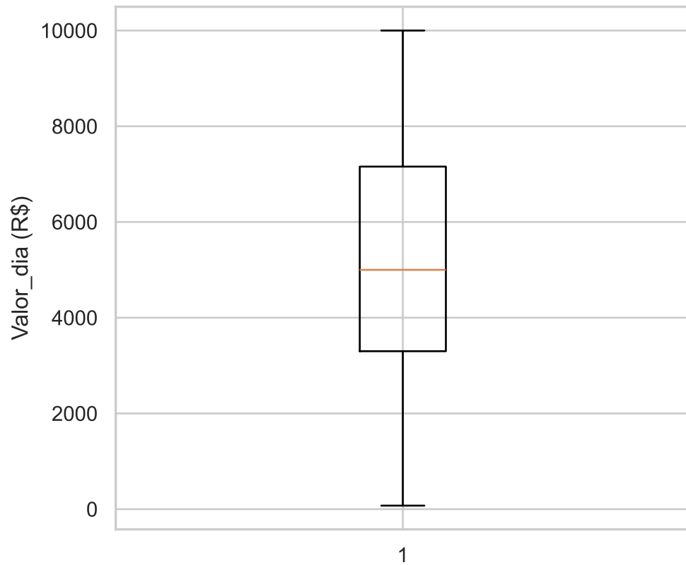
G1 — Pequenos Artistas — Valor_dia COM anomalias
