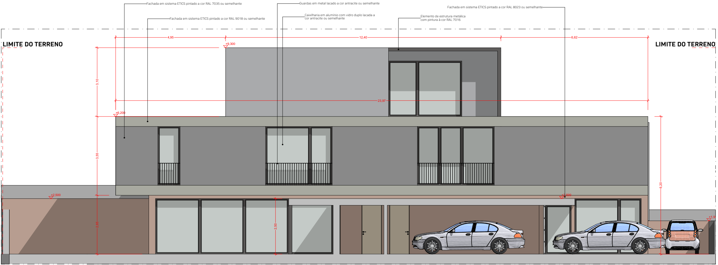
A-SUL - ALÇADO SUL
