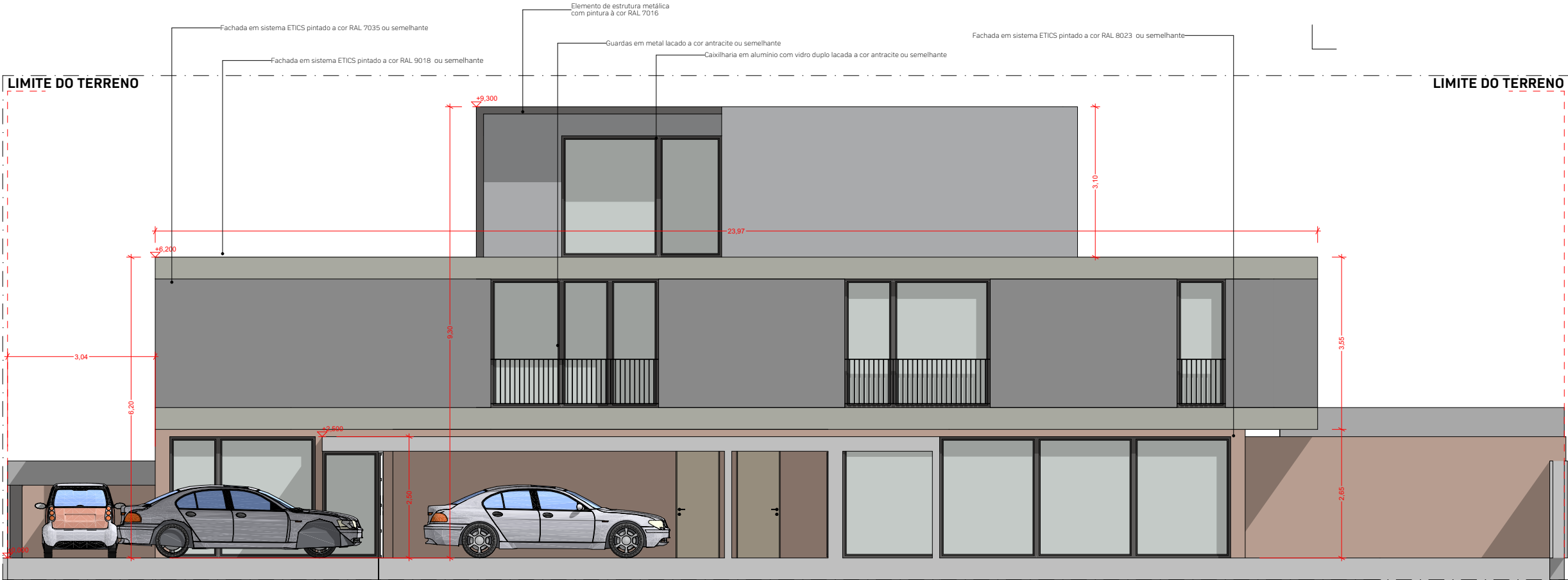
A-NOR - ALÇADO NORTE
