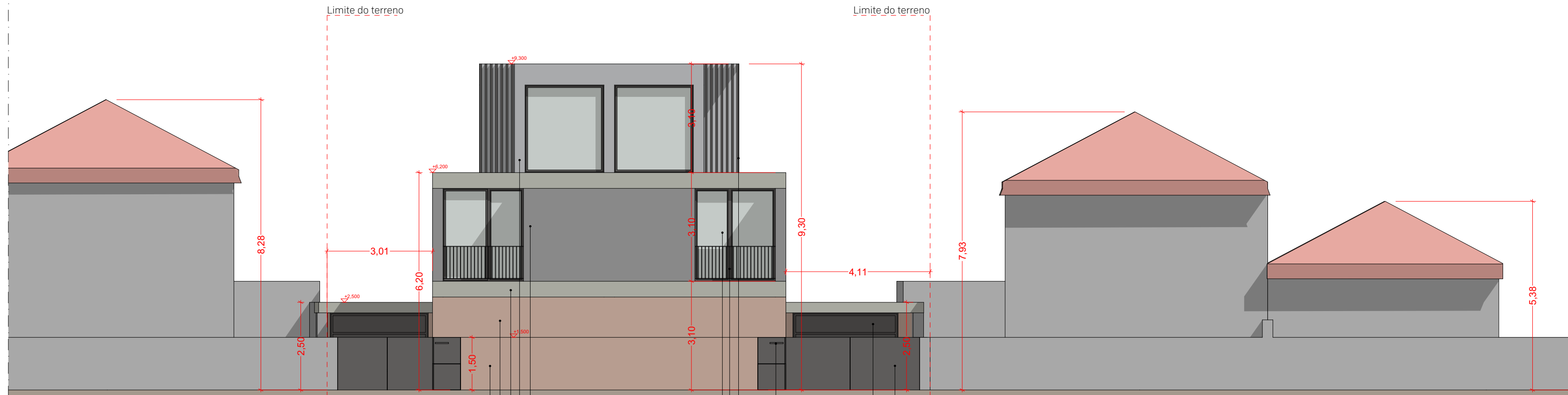
A-POE - ALÇADO POENTE
