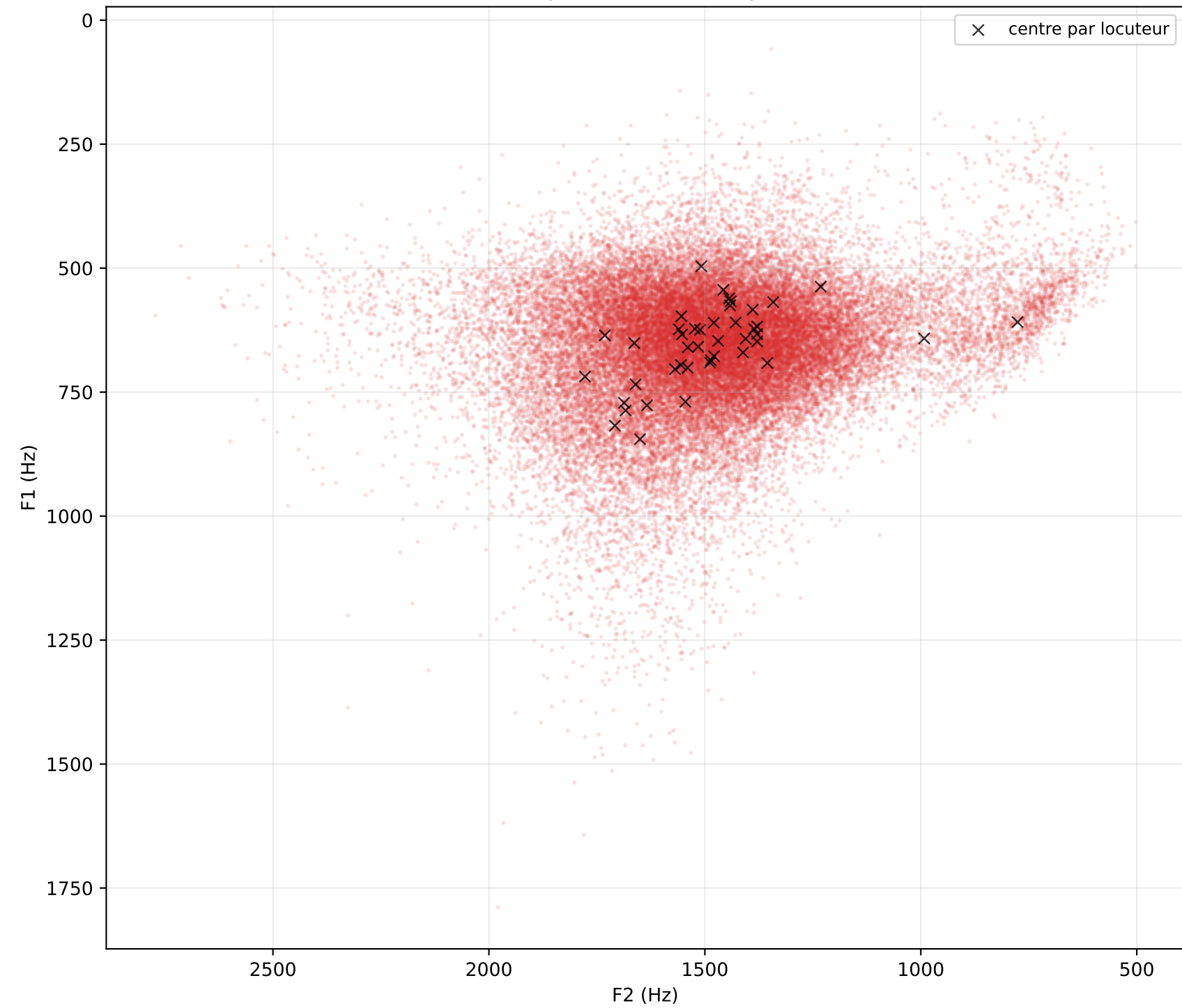
Tous les points F1-F2 — voyelle /a/
