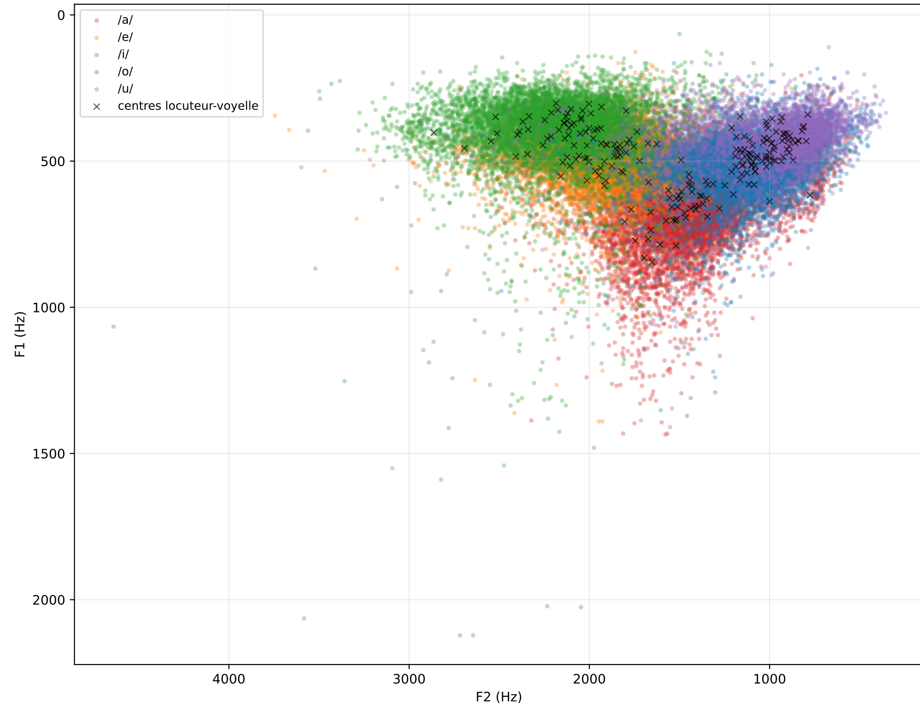
Tous les points F1-F2 — toutes les voyelles
