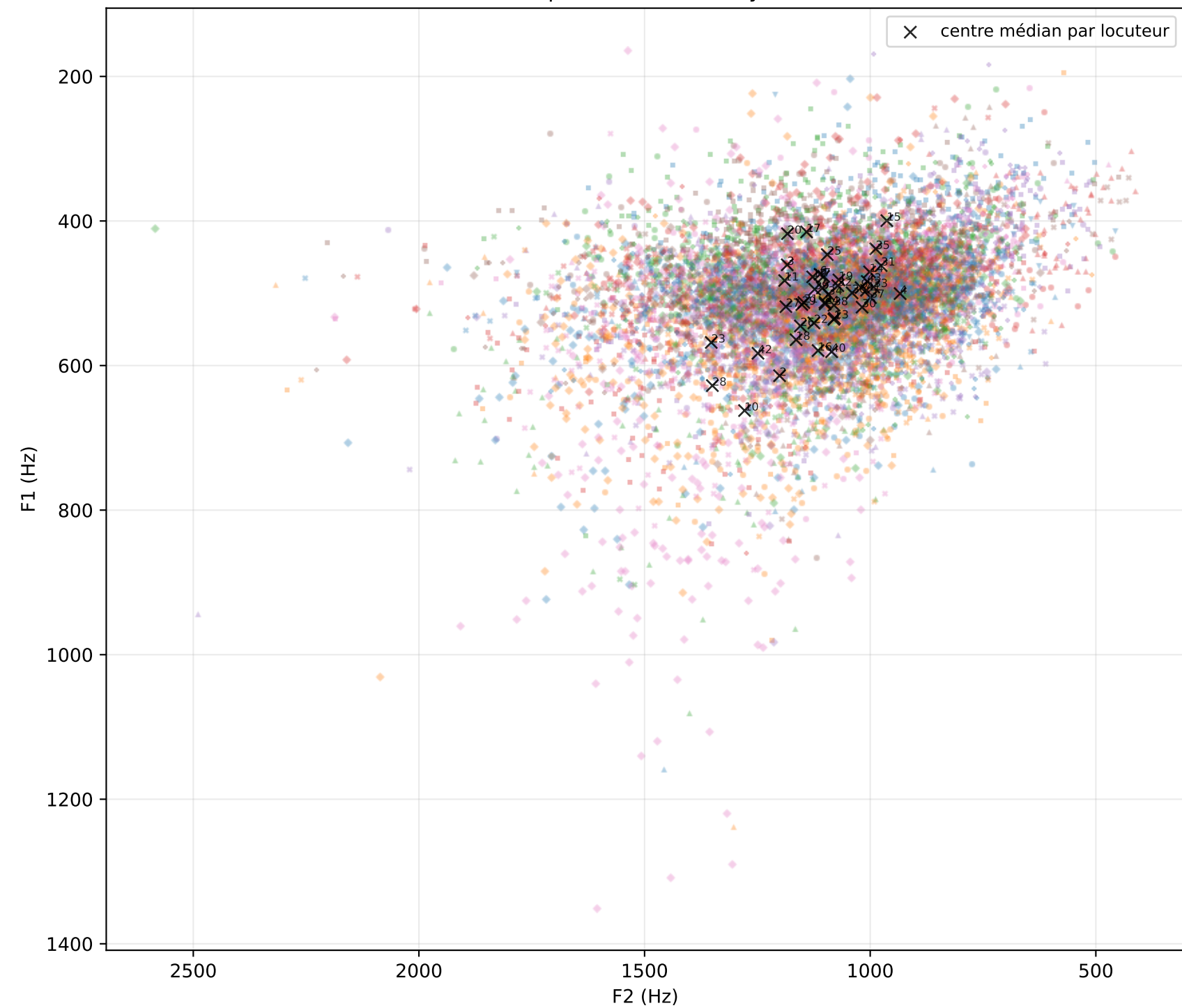
Tous les points F1-F2 — voyelle /o/
