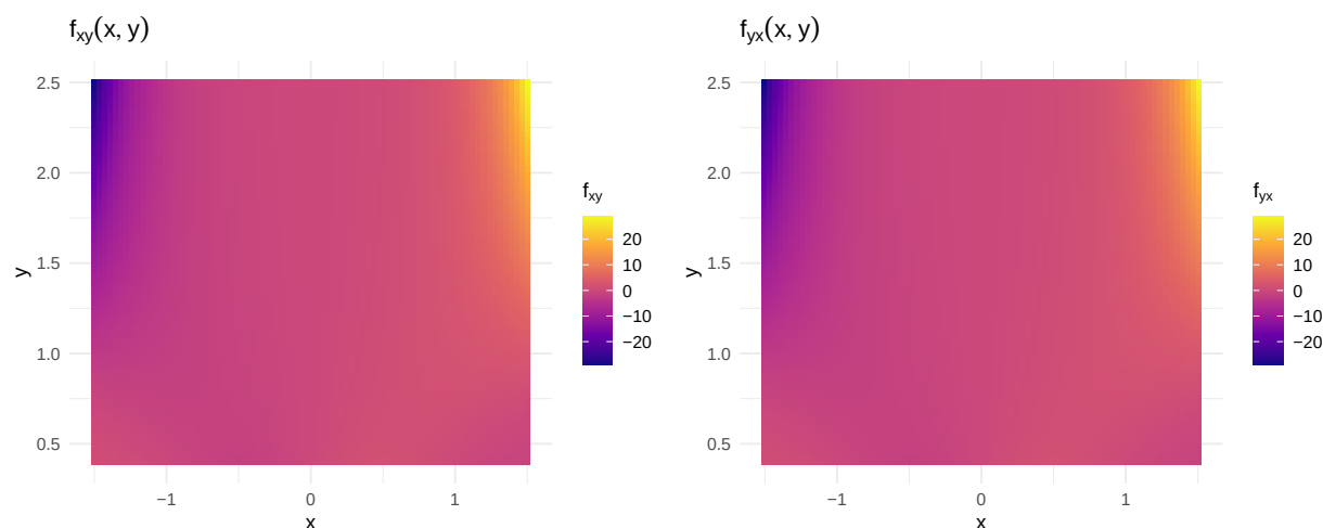
Figura 70: Verificação numérica das derivadas cruzadas de f(x, y) = y^{x^2} . Os dois painéis mostram f_{xy} e f_{yx} calculadas pela fórmula analítica 2xy^{x^2-1}[1 + x^2 \ln(y)] — visualmente idênticas, como exige Schwarz.
