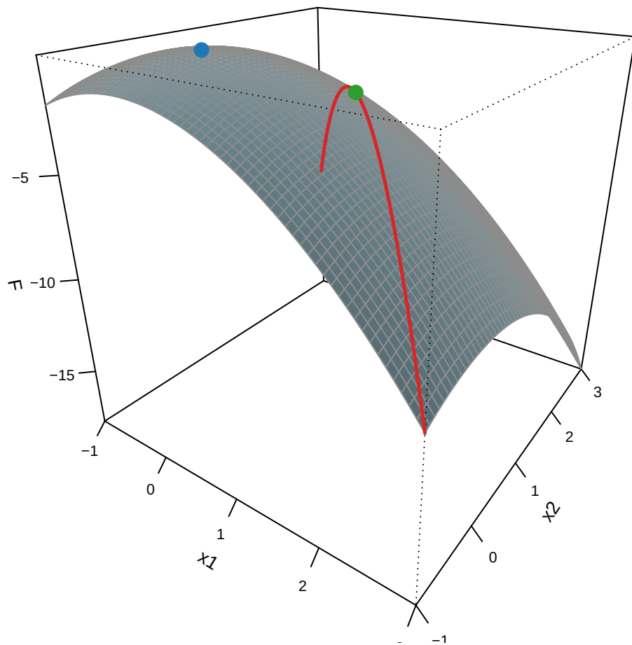
Figura 66: Vista 3D: superfície F(x_1, x_2) = -x_1^2 - x_2^2 (parabolóide invertido), restrição x_1 + x_2 = 2 traçada sobre a superfície (curva vermelha), ótimo irrestrito (0, 0, 0) em azul e ótimo restrito (1, 1, -2) em verde — ponto mais alto da curva vermelha.
