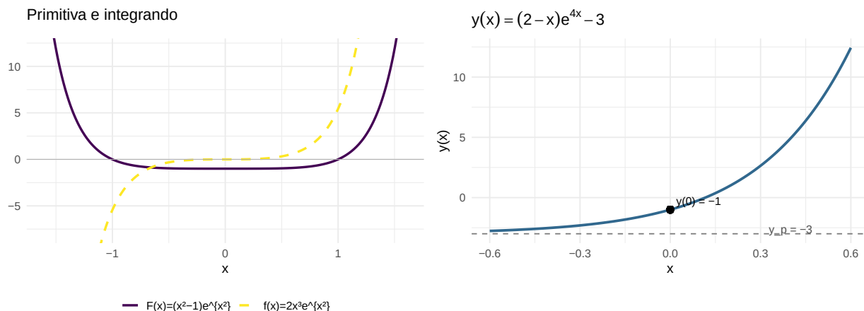
Figura 81: Esquerda: a primitiva (x^2 - 1)e^{x^2} (linha) e seu integrando 2x^3e^{x^2} (tracejado). Direita: solução da EDO y(x) = (2 - x)e^{4x} - 3 , com y(0) = -1 marcado; o fator (2 - x)e^{4x} domina o crescimento.
