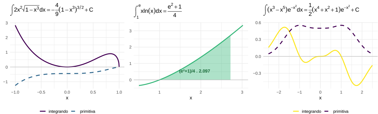
Figura 45: Verificação numérica das integrais do Teste 3 (2026). Esquerda: integrando 2x^2\sqrt{1-x^3} e sua primitiva -\frac{4}{9}(1-x^3)^{3/2} . Centro: integral definida \int_1^e x \ln(x) dx = \frac{e^2+1}{4} representada como área sombreada. Direita: integrando (x^3-x^5)e^{-x^2} e sua primitiva \frac{1}{2}(x^4+x^2+1)e^{-x^2} .
