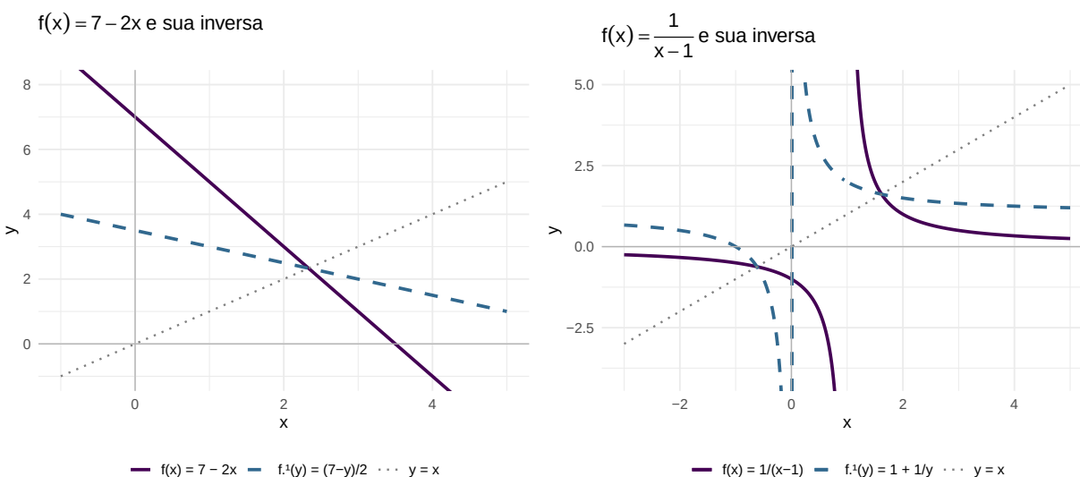
Figura 35: Gráficos de f e f^{-1} refletidos em torno de y = x . Exemplos: f(x) = 7 - 2x (esquerda) e f(x) = 1/(x-1) (direita).
