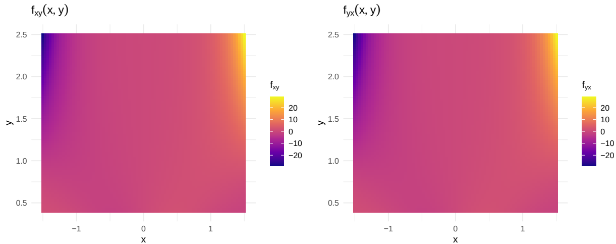
Figura 70: Verificação numérica das derivadas cruzadas de f(x, y) = y^{x^2} . Os dois painéis mostram f_{xy} e f_{yx} calculadas pela fórmula analítica 2x y^{x^2-1} [1 + x^2 \ln(y)] — visualmente idênticas, como exige Schwarz.
