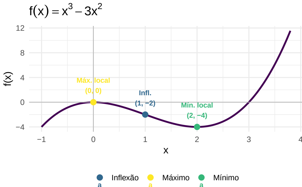
Figura 13: Análise completa de f(x) = x^3 - 3x^2 : máximo local, mínimo local e ponto de inflexão
