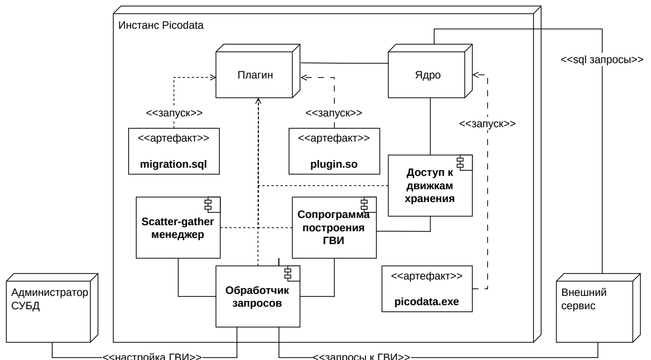
Рисунок 9 — Диаграмма развертывания плагина в рамках одного узла СУБД Picodata
