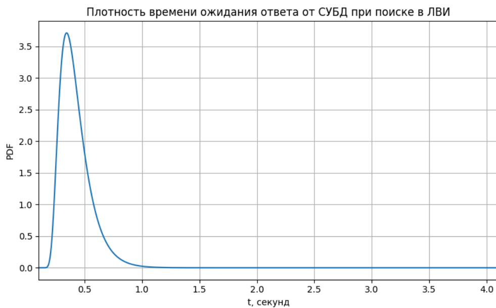
Рисунок 11 — Плотность вероятности времени ожидания ответа от СУБД при поиске в ЛВИ
