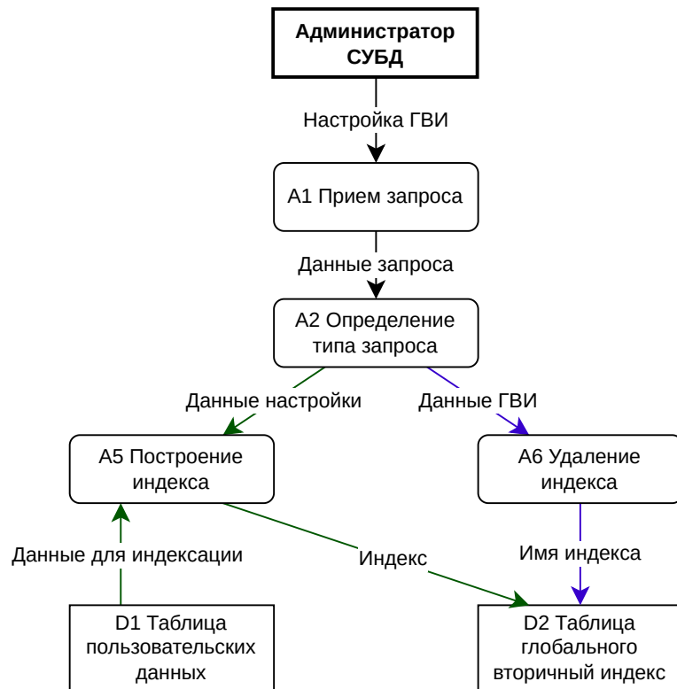
Рисунок 8 — Диаграмма потоков данных использования плагина ГВИ администратором СУБД
