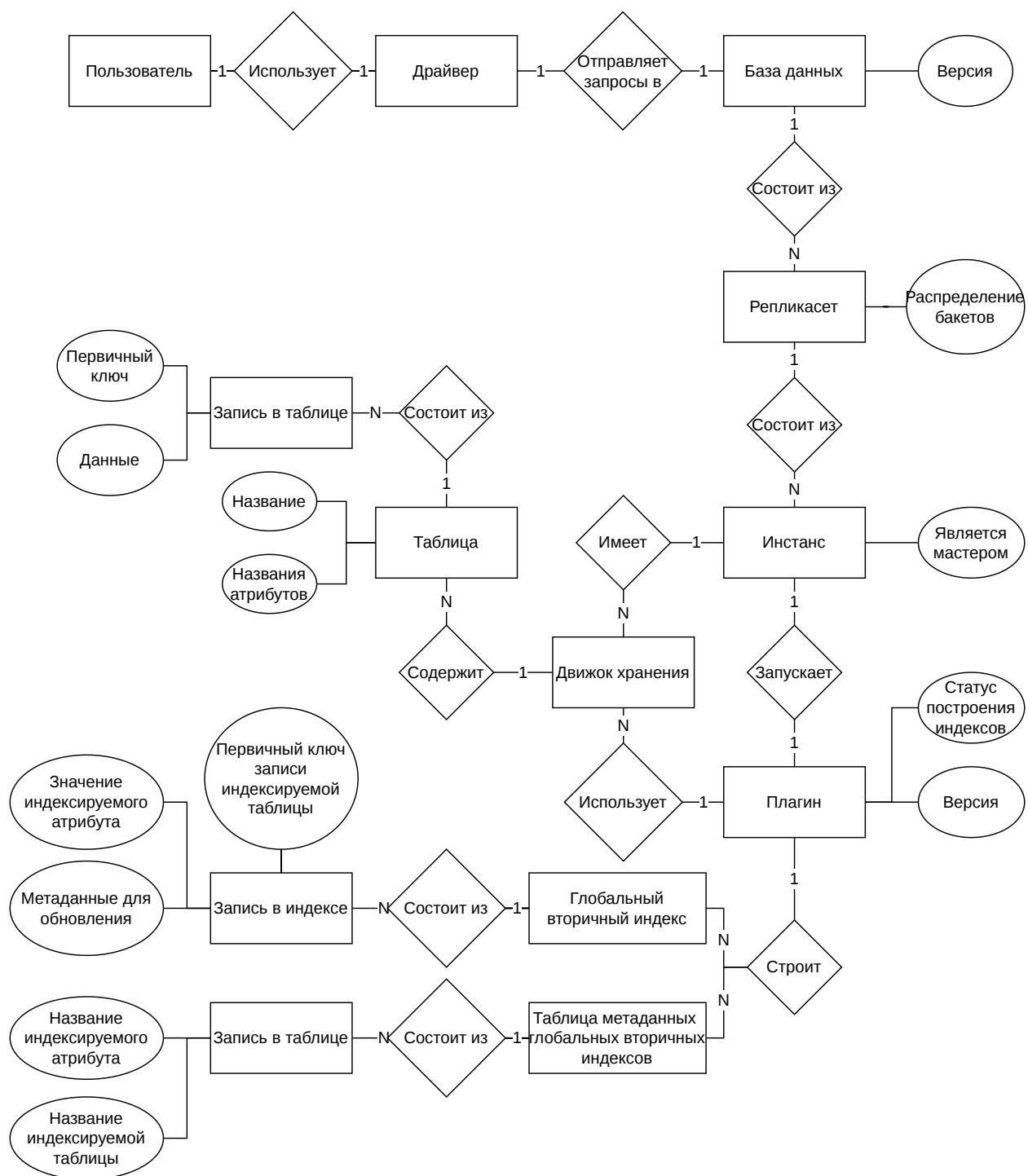
Рисунок 1 — ER-диаграмма
