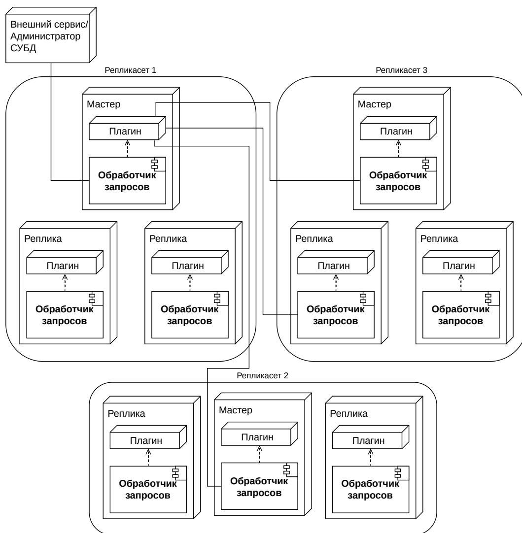
Рисунок 11 — Диаграмма развертывания плагина в рамках кластера СУБД Picodata
