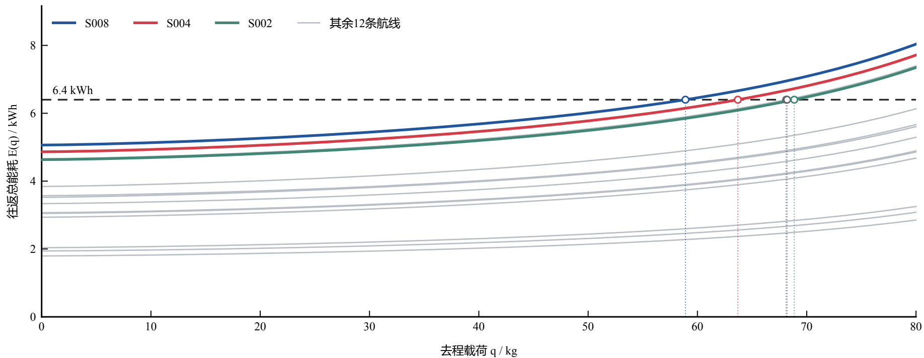
(a) 能耗—载荷关系
