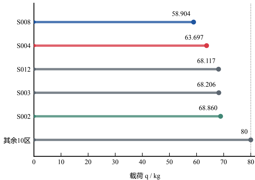
(c) 可行载荷区间
