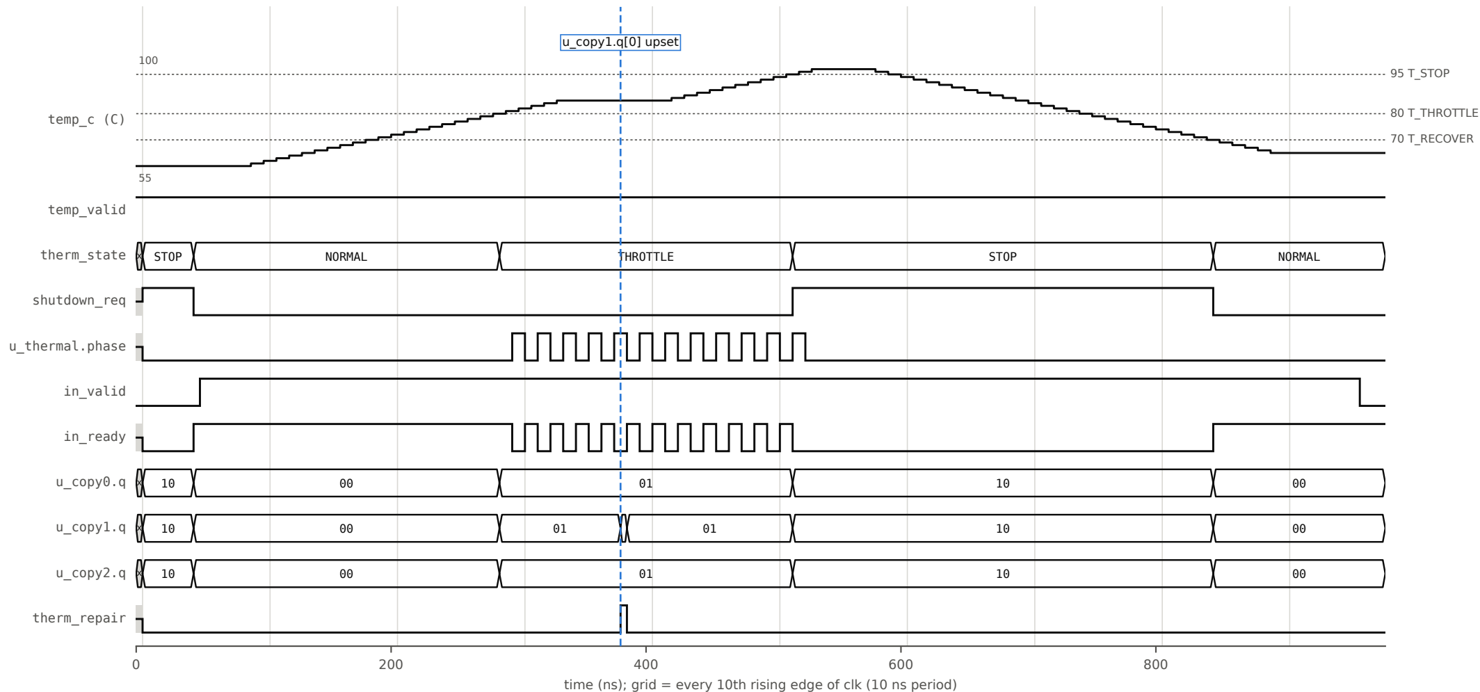
(d) thermal ramp 60 -> 85 -> 97 -> 65 C, one reading per cycle, temp_valid = 1
