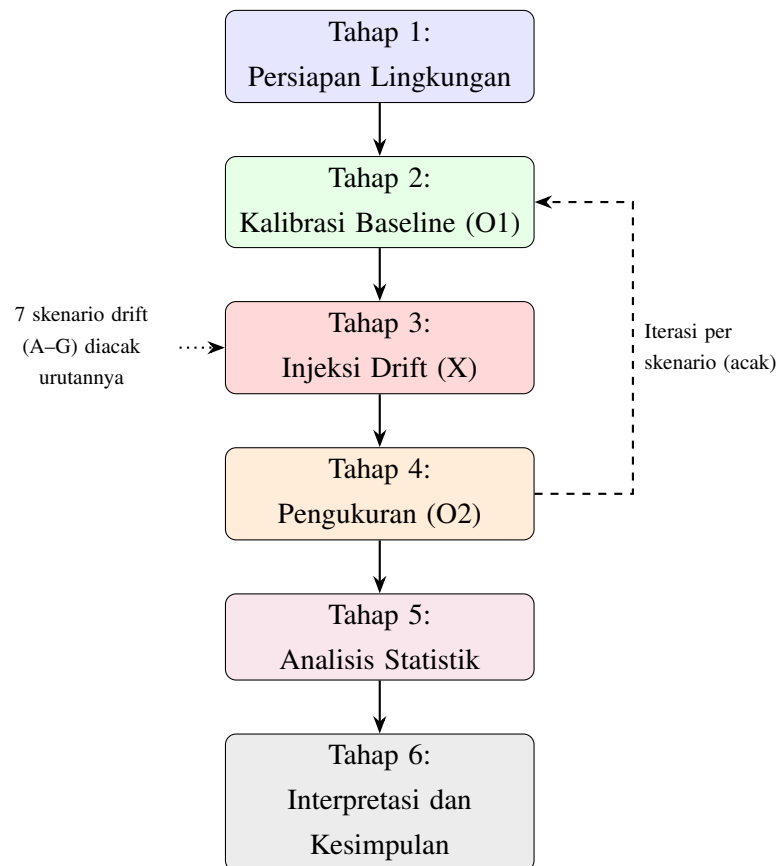
Gambar 3.2: Bagan alir eksperimen: tahapan penelitian dari persiapan hingga interpretasi. Iterasi per skenario menunjukkan pengulangan acak dari baseline hingga pengukuran untuk setiap skenario drift.
