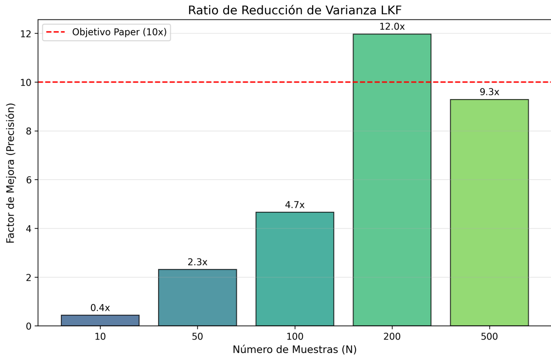
Figura 7: Ratio de Reducción de Varianza (LKF). Resultado agregado de 100 corridas Monte Carlo . El filtro LKF logra una reducción de varianza de 12,0 \times para N = 200 muestras, cumpliendo el objetivo de 10 \times . El AKF supera al LKF en un 12,5 % (13,5 \times vs 12,0 \times ) pero con 35 % más de overhead computacional.
