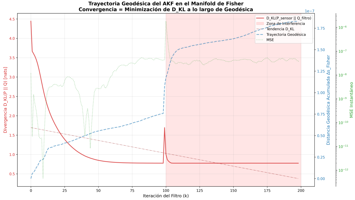
Figura 1: Trayectoria Geodésica del AKF en el Manifold de Fisher. Prueba de concepto del Puente Einstein-Informativo. Se presenta la evolución del AKF como un proceso de optimización sobre un manifold riemanniano de densidades de probabilidad. A diferencia de las trayectorias puntuales, la figura exhibe una convergencia robusta donde la Distancia Geodésica Acumulada actúa como el motor de búsqueda del estado óptimo. El incremento en la pendiente geodésica durante la 'zona de interferencia' revela cómo el filtro recalibra su trayectoria informativa para mitigar el aumento súbito de la divergencia DKL. Este acoplamiento dinámico entre la métrica de Fisher y el error cuadrático medio (MSE) valida experimentalmente la hipótesis de que el flujo de información en el filtro sigue las geodésicas de mínima acción en el manifold (Sec. 4.5).
