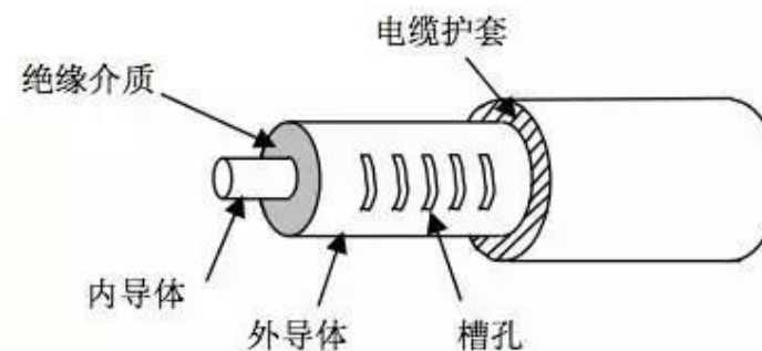
同轴电缆
