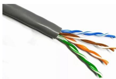
4对双绞线 构成网线
