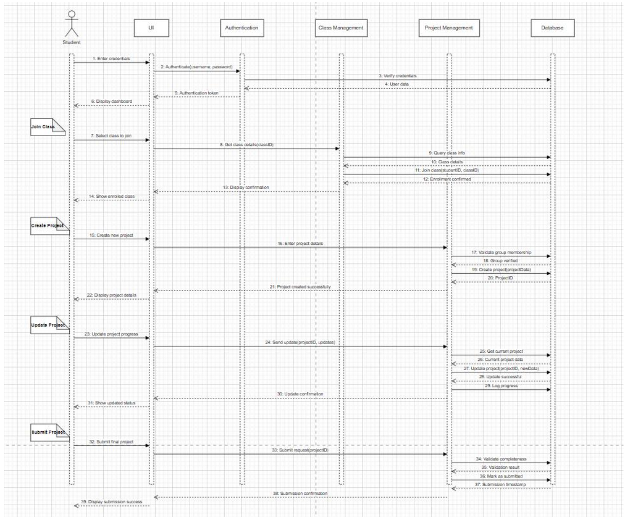
Fig. 4.3 Sequence diagram of Mini Project
