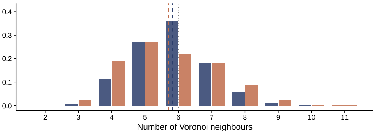
Velavadar_LEK2
