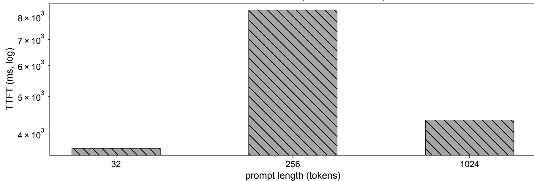
LLM — Llama-3.2-1B (LiteRT-LM, TTFT)
