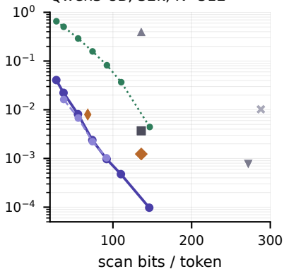
Qwen3-8B, 32k, K=512
