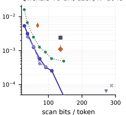
Qwen2.5-7B-1M, 128k, K=2048
