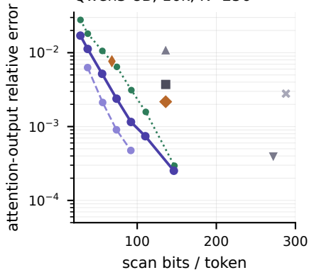
Qwen3-8B, 16k, K=256
