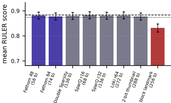
Qwen3-8B, 32k, K=128
