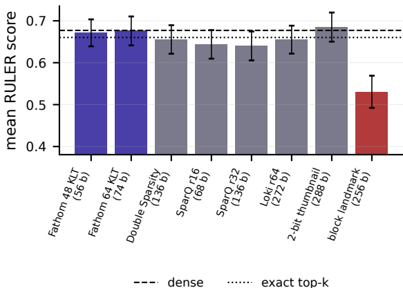
Qwen2.5-7B-1M, 128k, K=128
