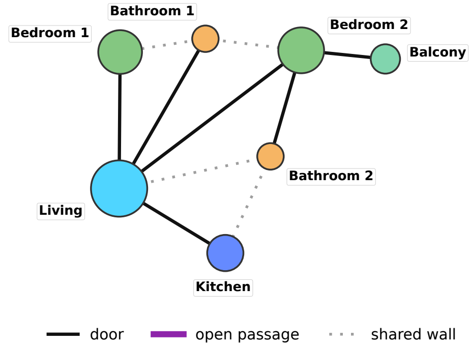
(d) M4 typed bubble diagram
