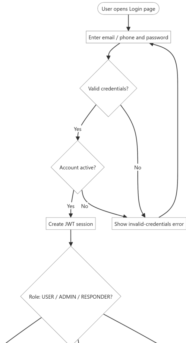
Flowchart 4.2.1: Login
