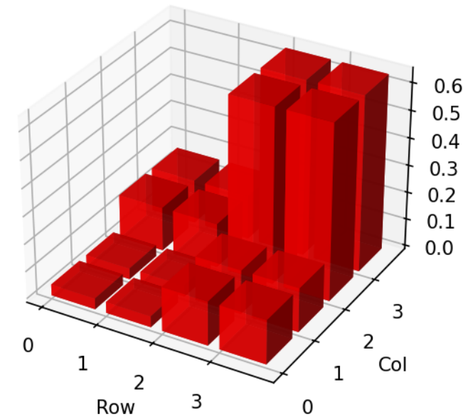
QAOA p=1 gamma=1.0 beta=0.8
