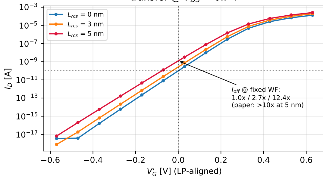
transfer @ V_{DS} = 0.7 V
