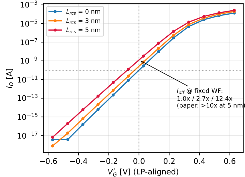
transfer @ V_{DS} = 0.7 V
