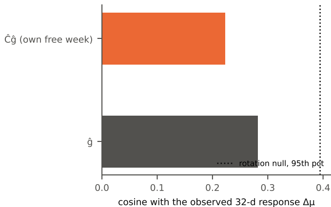
(d) P4: D = -0.060 [-0.164, 0.056]
