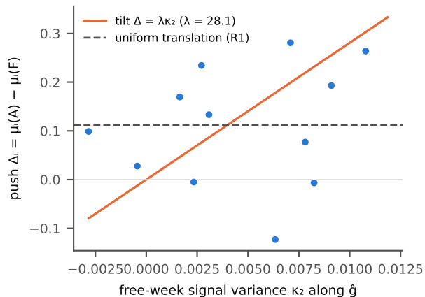
(d) P4: D = -0.060 [-0.164, 0.056]
