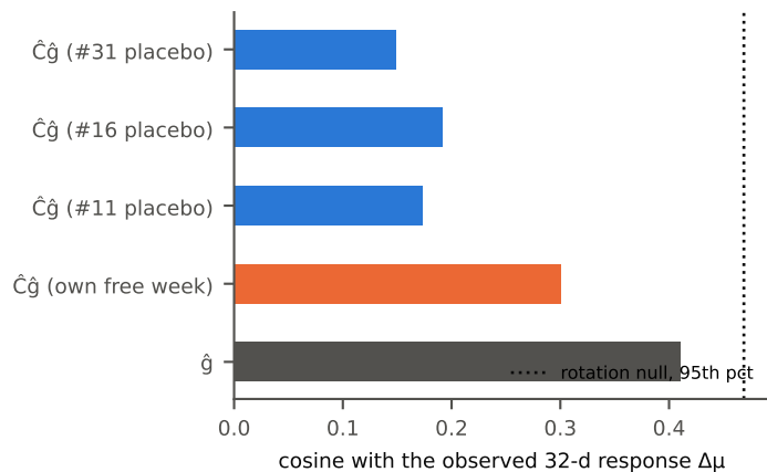
(d) P4: D = -0.110 [-0.282, 0.085]
