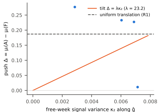
(d) P4: D = -0.110 [-0.282, 0.085]
