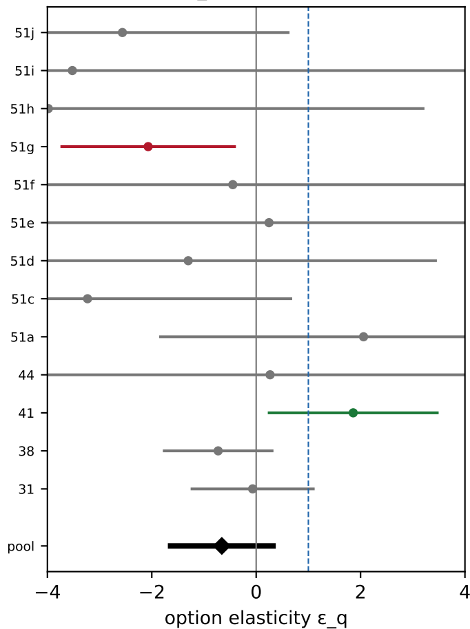
work: \epsilon_q per unit (95% CI)
