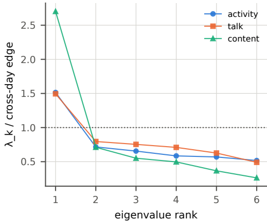
G18 spectra (18)
