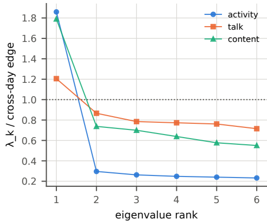
G23 spectra (23)
