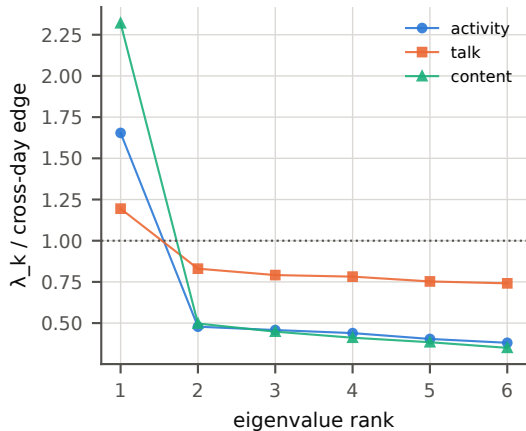
G30 spectra (30)
