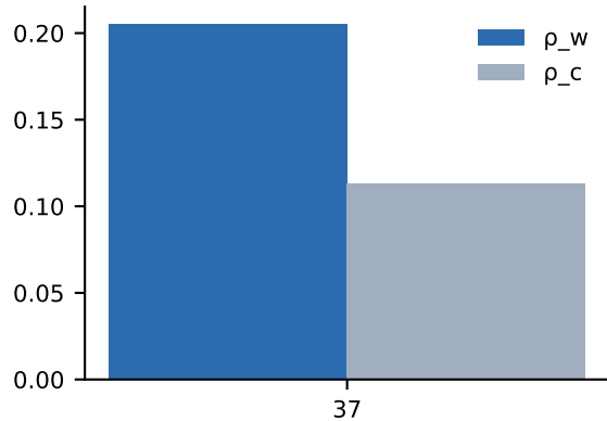
G37: C_B 0.55 (p 0.080)
