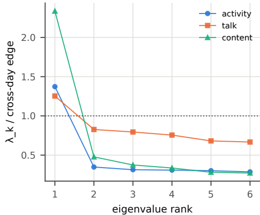
G26 spectra (26)
