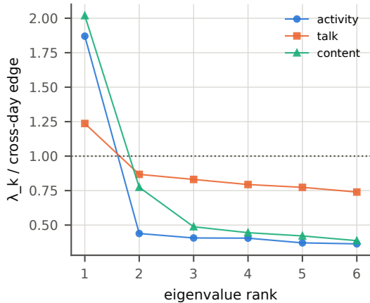
G35 spectra (35)
