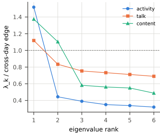
G44 spectra (44)
