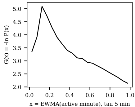
(d) betaJ0 0.15; p(valley) 1.00
