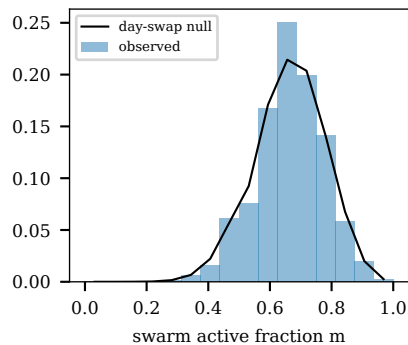
(d) betaJ0 0.15; p(valley) 1.00
