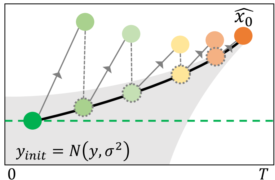
(d) Inference process of proposed DDTSE-only mode
