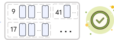
Correct Traj.
