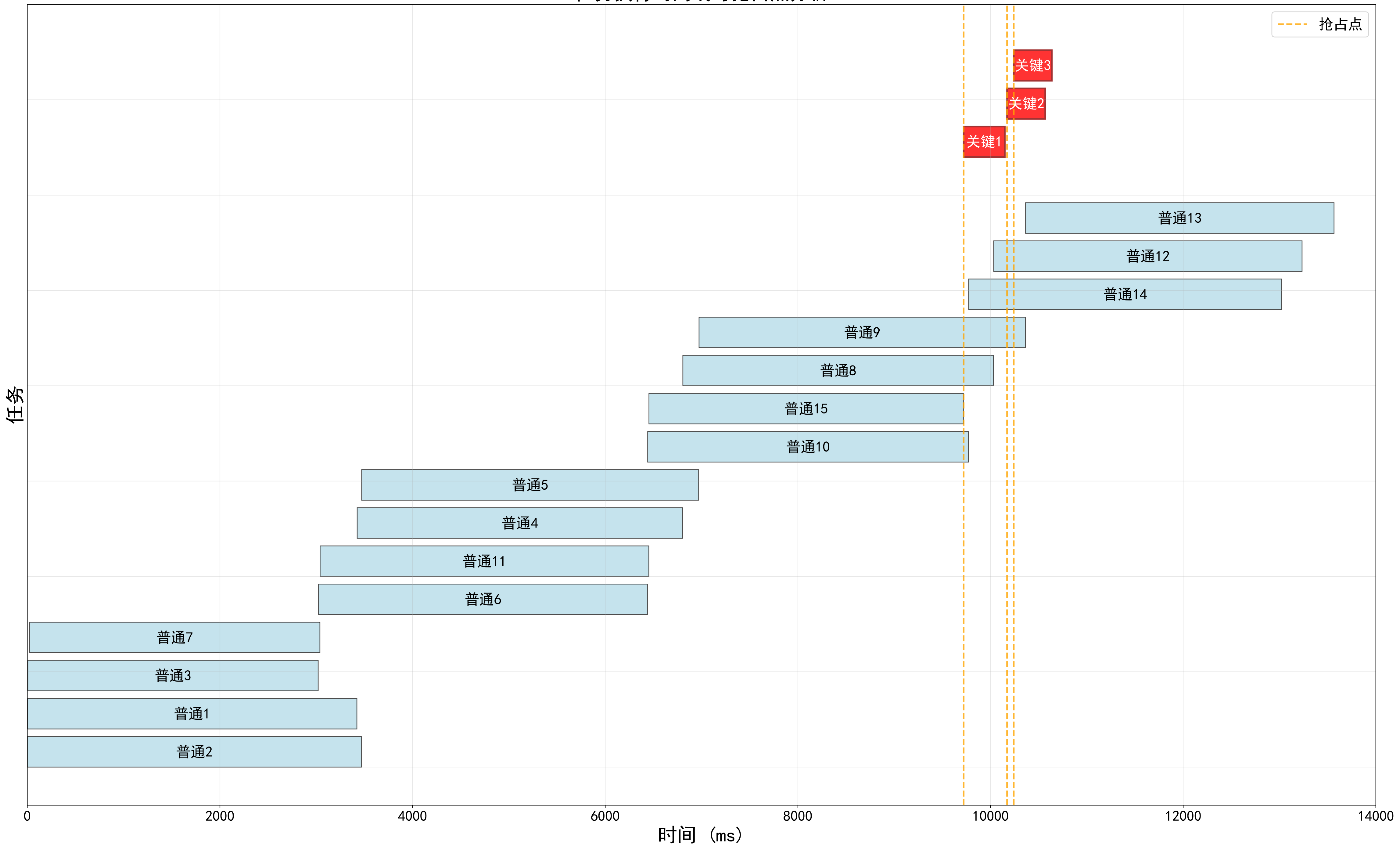
任务执行时间线与抢占点分析
