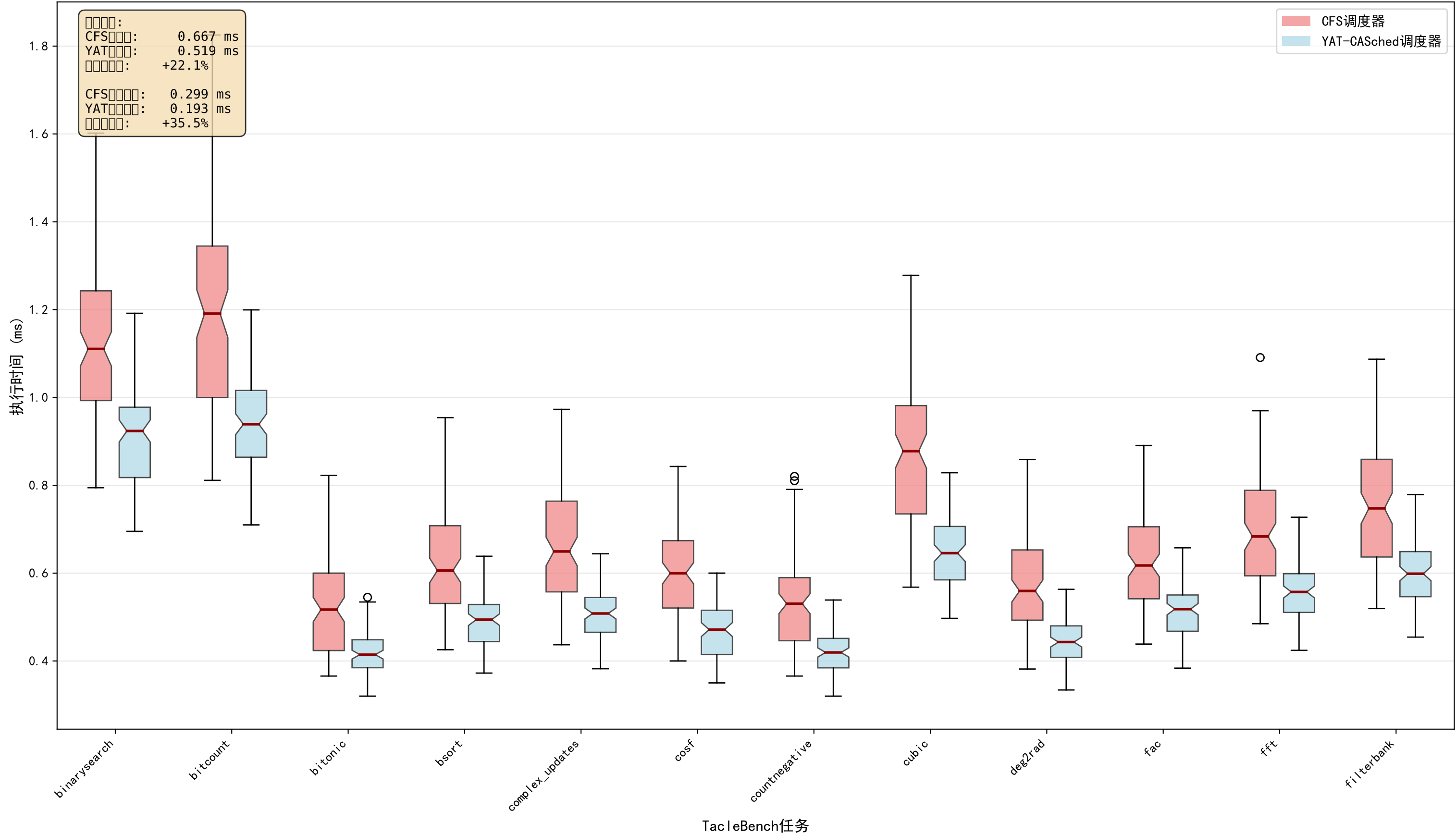
Tac leBench任务集执行时间分布对比 (CFS vs YAT-CASched)
