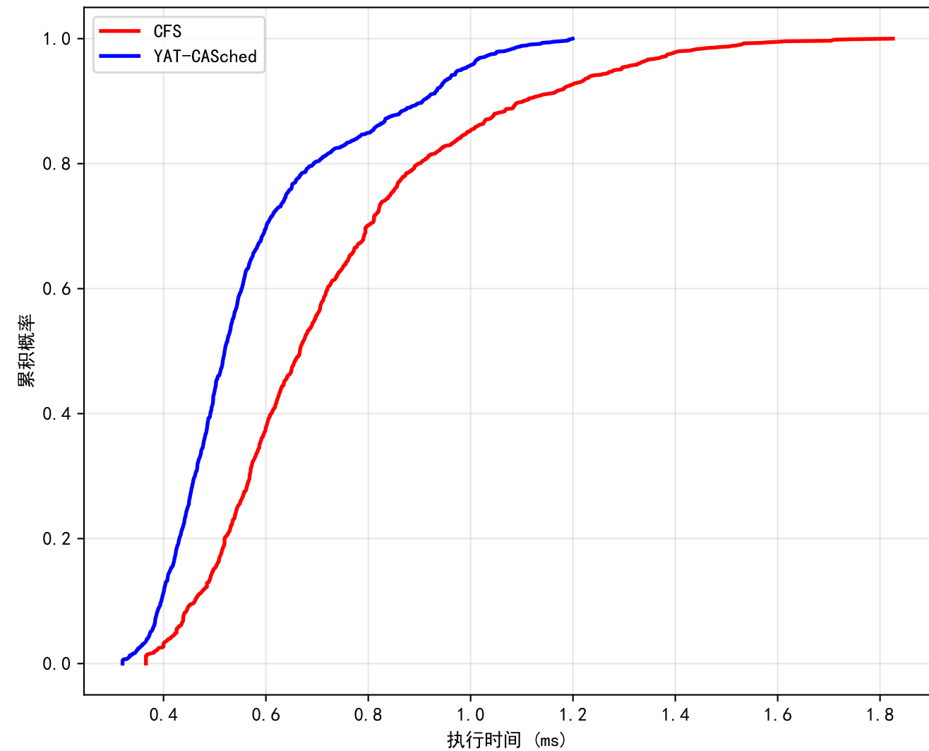
累积分布函数对比
