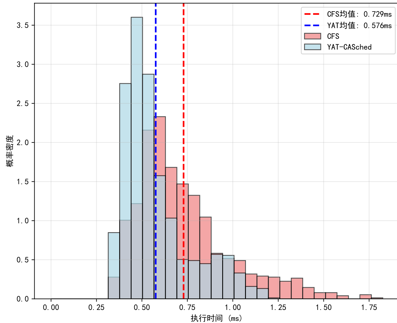
总体执行时间分布对比
