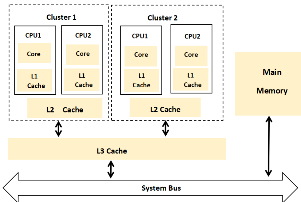
图 6: 多核系统缓存层次结构
