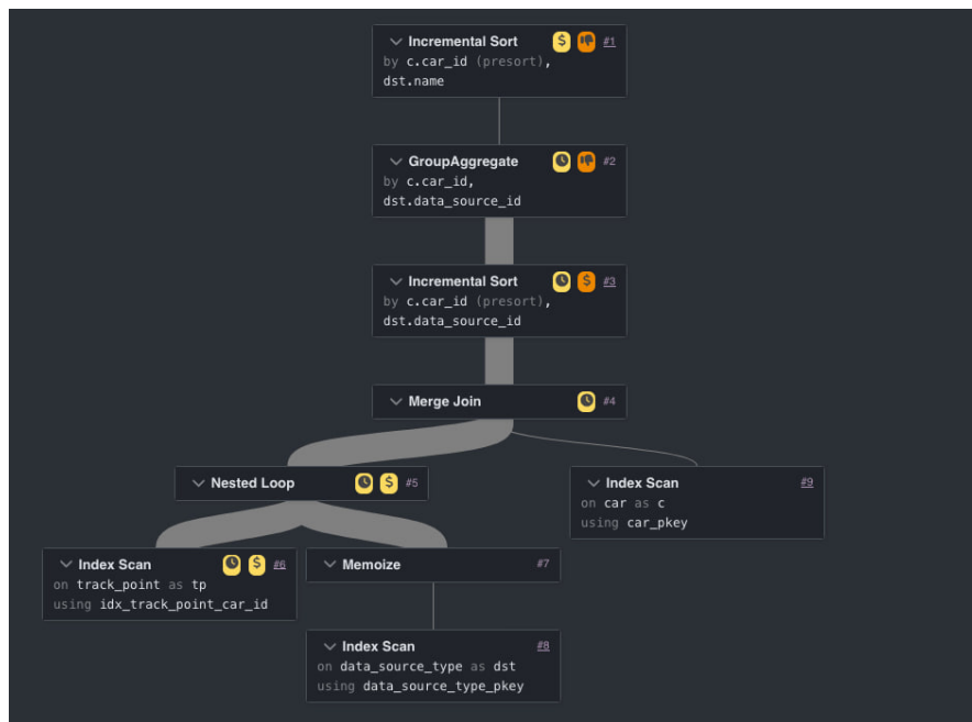
Рис. 27: План выполнения запроса 8
