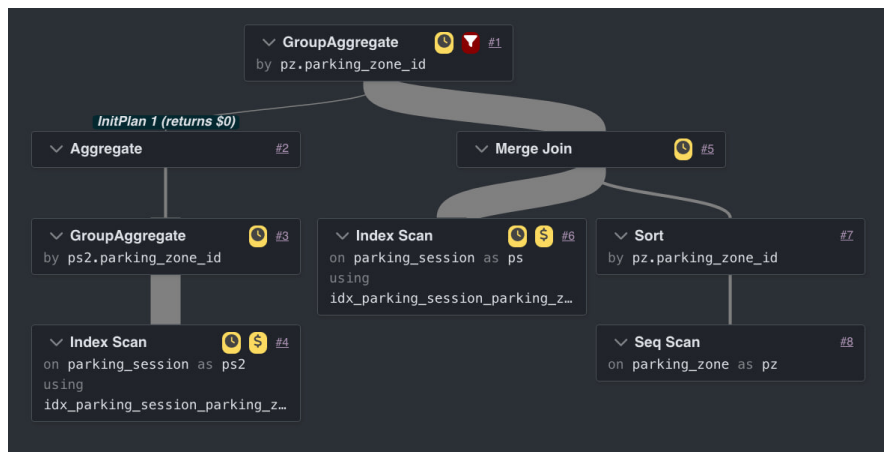
Рис. 16: План выполнения запроса 4 (макс)
