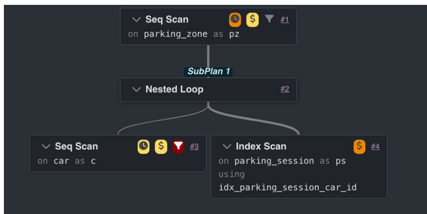
Рис. 25: План выполнения запроса 7
