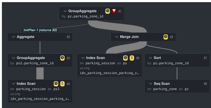
Рис. 18: План выполнения запроса 4 (мин)
