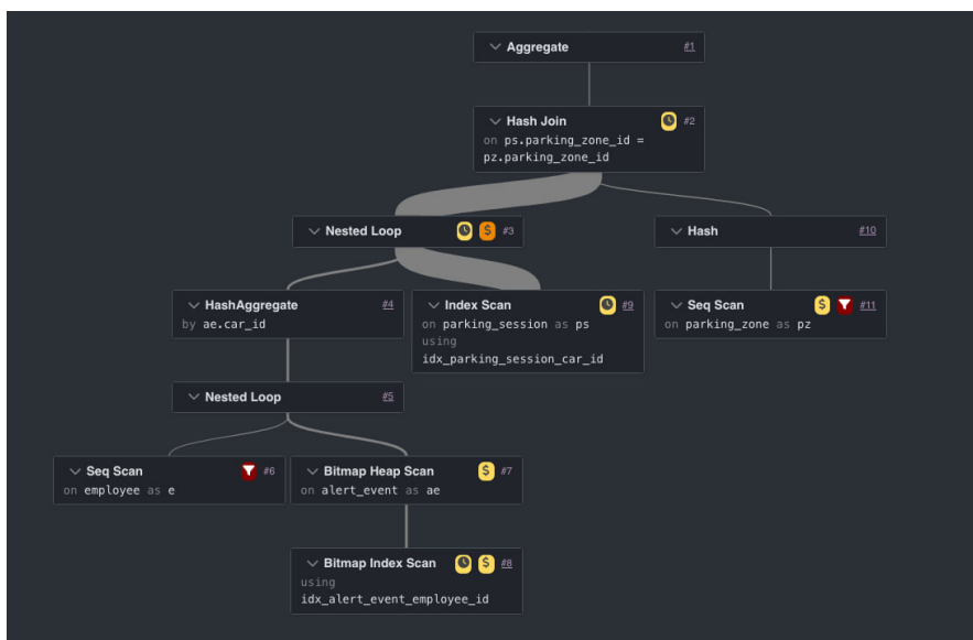
Рис. 11: План выполнения запроса 2
