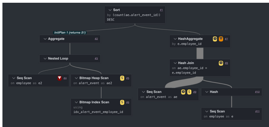
Рис. 23: План выполнения запроса 6
