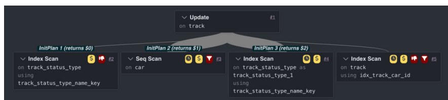
Рис. 29: План выполнения запроса 9
