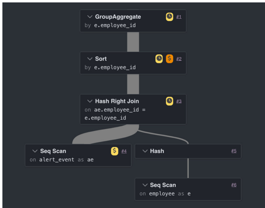
Рис. 13: План выполнения запроса 3
